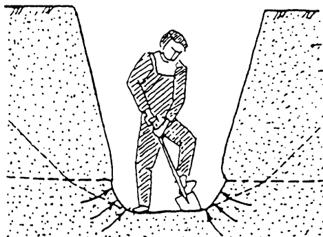
Mynd 5 Dæmi um hættulegar aðstæður. Skurðurinn er orðinn dýpri en grunnvatnsstaðan og lítil halli er á hliðunum.
